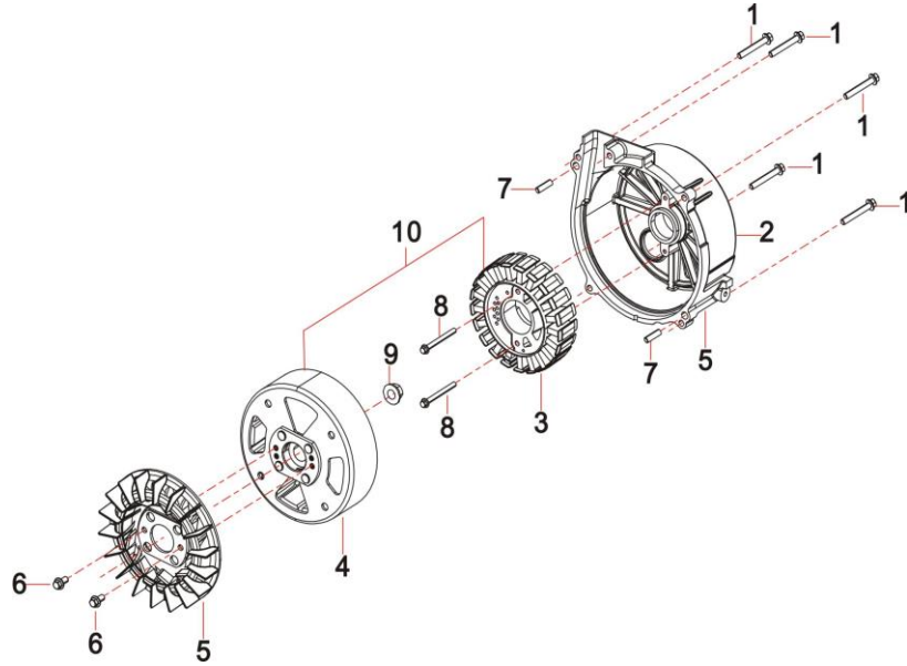
FIG.7 ROTOR/STATOR 电机组件 (F63)
